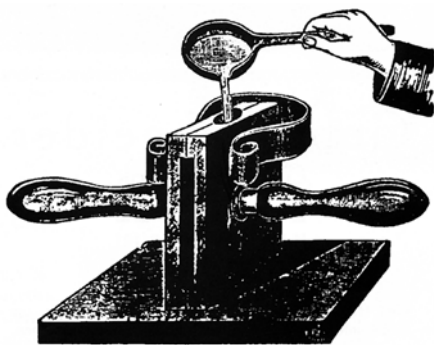
Støbeform med fjeder og træhåndtag fyldes med flydende metal fra støbeskeen
